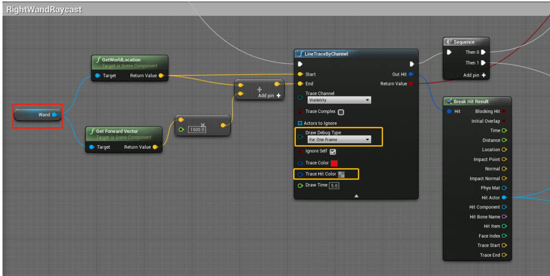
图 3.14 右手柄射线检测
