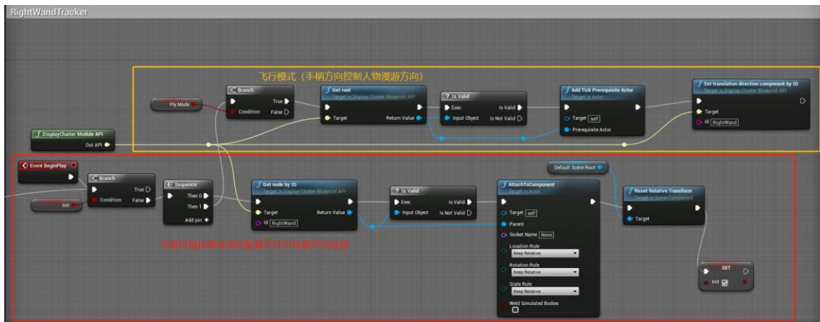
图 3.11 右手柄追踪与控制
