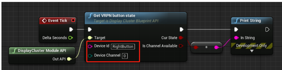
图 2.7 获取右手柄 VRPN Trigger 按键
