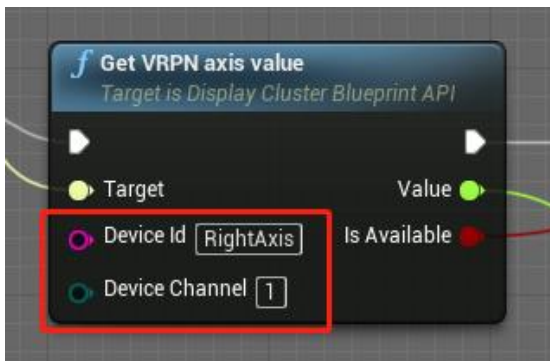
图 3.7 获取右手柄摇杆纵轴
