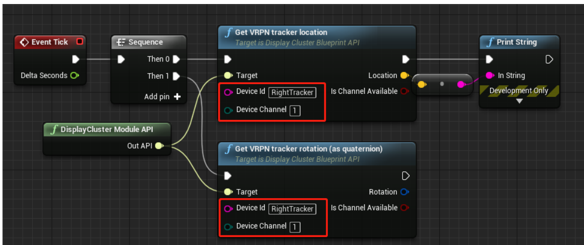
图 2.5 获取右手柄 VRPN 追踪
